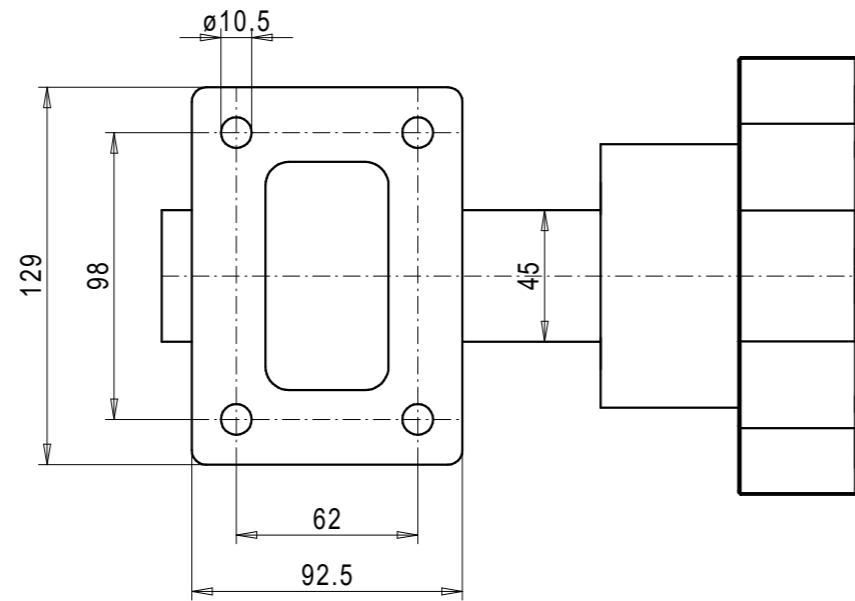
View A-A
